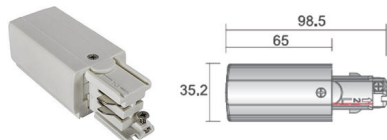
Napajec levý
