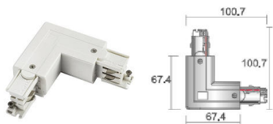
Roh 90° levý
