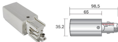
Napajec pravý
